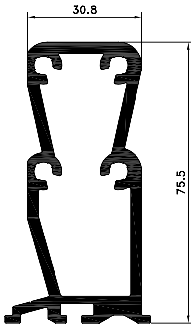
REF. 11050 Perfil tope escuadra APT 050
