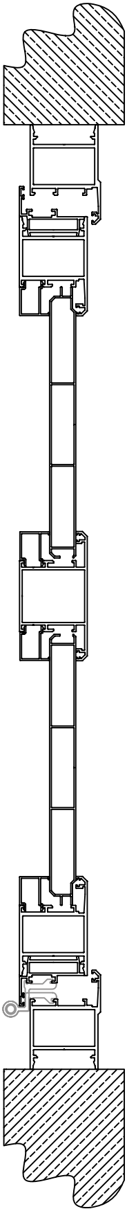
Puerta de paso. Bisagra CE. Travesaño interior.
