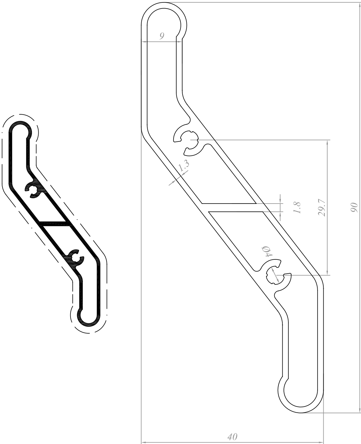
REF. 1102090 Lama ventilada CÓD. TS 2090
