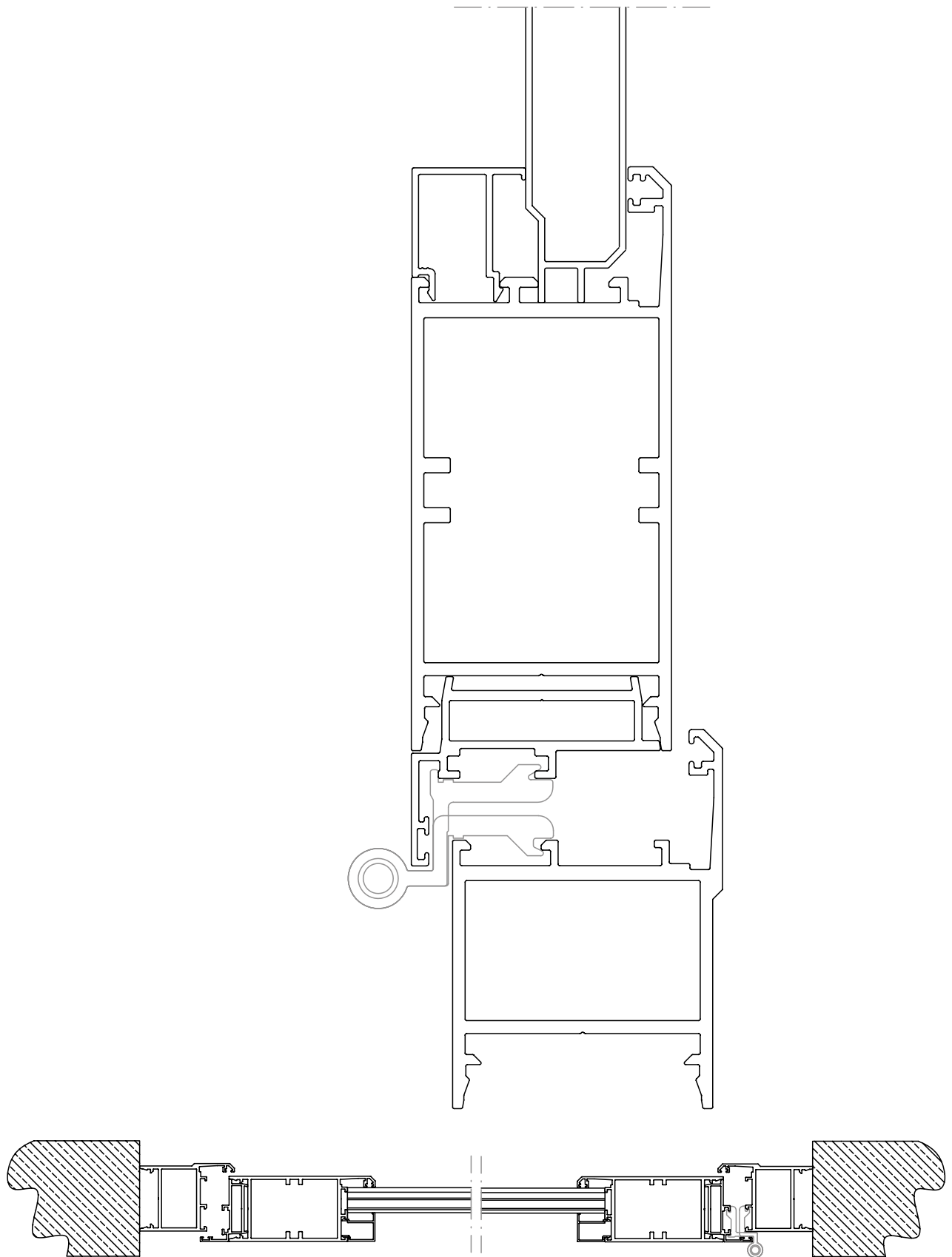
Puerta de paso. Bisagra CE
