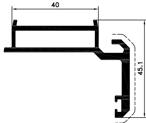
REF. 11006 Batiente puerta 2 hojas APT 006
